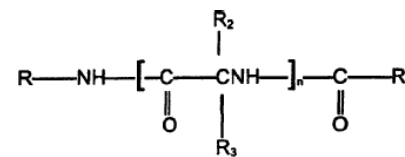
Fórmula (Ia)
